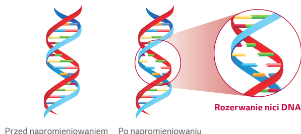
Zniszczenie sekwencji (łańcucha) nukleotydów
