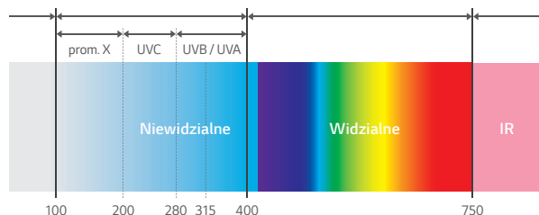
Spektrum i rodzaje promieniowania elektromagnetycznego
